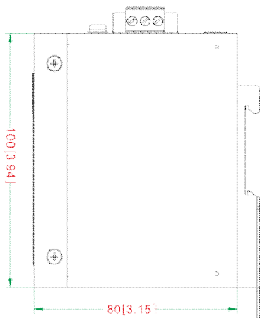
左侧视图
